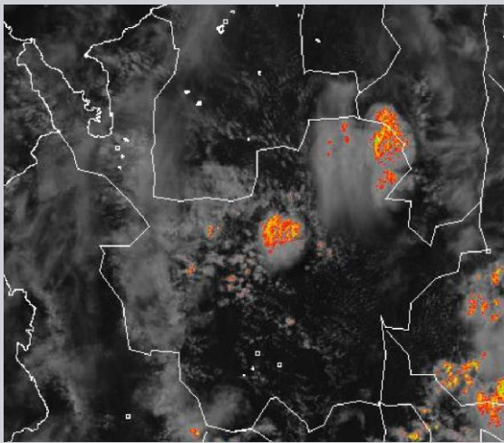
Imagen Canal Visible - IDEAM – junio 16 de 2016 – Hora 2:15 p.m. HLC.
