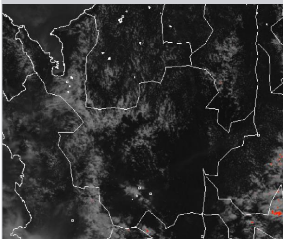
Imagen Canal Visible - IDEAM – junio 17 de 2016 – Hora 12:15 a.m. HLC.
