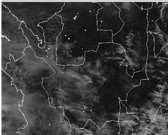
Imagen Canal Visible - IDEAM – julio 12 de 2016 – Hora 12:15 a.m. HLC.
