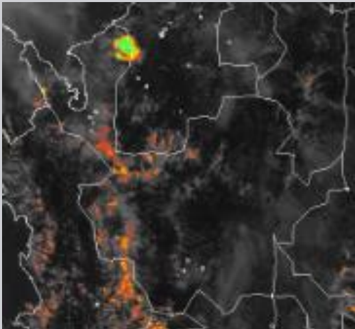
Imagen Canal Visible - IDEAM – julio 14 de 2016 – Hora 12:15 p.m. HLC.
