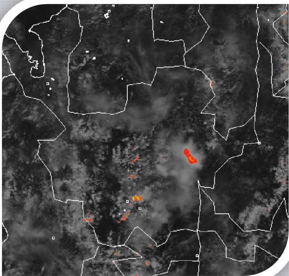
Nubosidad representada en la imagen satelital. Canal Visible - IDEAM – octubre 23 de 2016 – Hora 1245 p.m. HLC.
