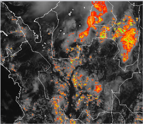
Nubosidad representada en la imagen satelital. Canal Visible - IDEAM – octubre 13 de 2016 – Hora 12:45 p.m. HLC.
