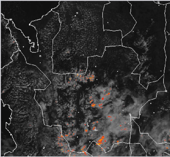
Nubosidad representada en la imagen satelital. Canal Visible - IDEAM – Febrero 12 de 2017 – Hora 12:15 p.m. HLC.
