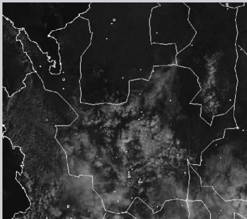
Nubosidad representada en la imagen satelital. Canal Visible – GOES- IDEAM – febrero 24 de 2017 Hora 12:15 p.m. HLC.
