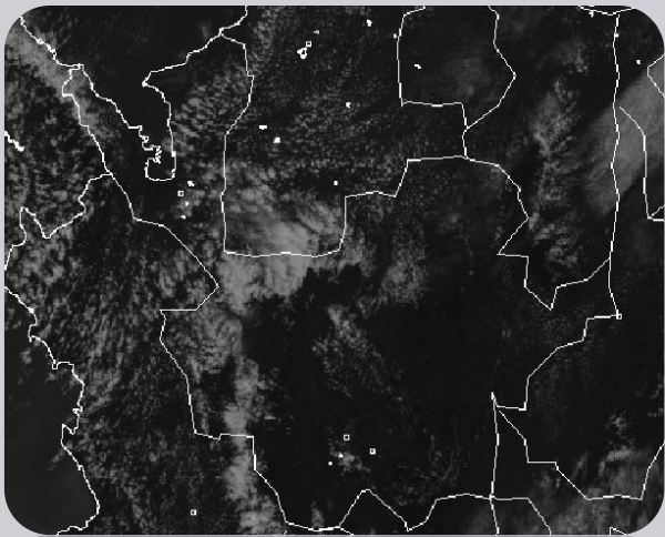
Nubosidad representada en la imagen satelital. Canal Visible – GOES - IDEAM Abril 15 de 2017 – Hora 1:15 p.m. HLC.
