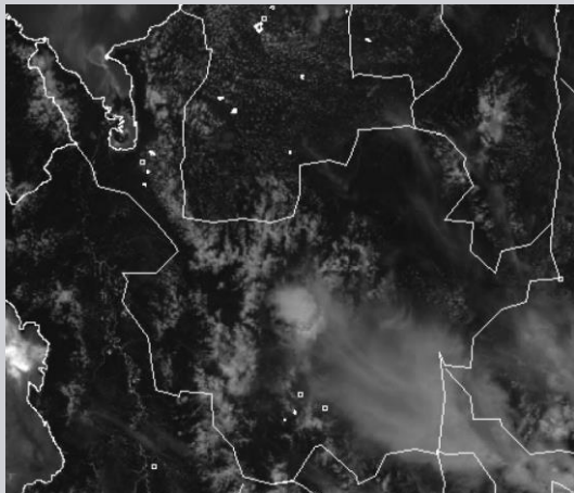
Nubosidad representada en la imagen satelital. Canal Visible – GOES- IDEAM – Abril 21 de 2017 Hora 12:15 p.m. HLC.
