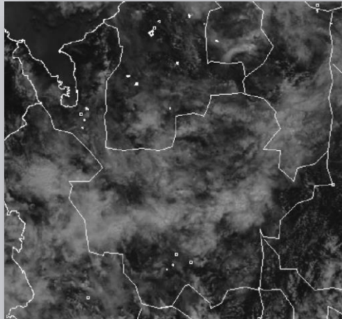
Nubosidad representada en la imagen satelital. Canal Visible – GOES- IDEAM – Junio 9 de 2017 Hora 11:45 a.m. HLC.
