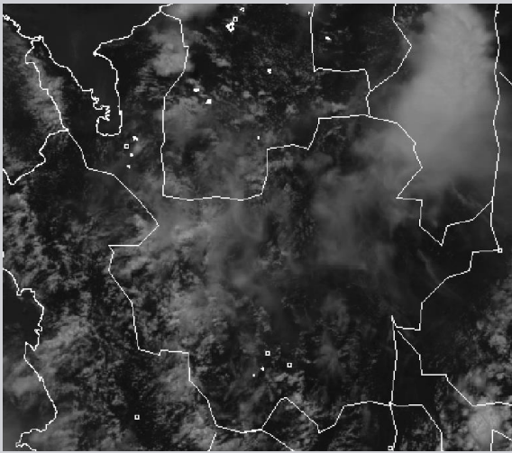
Nubosidad representada en la imagen satelital. Canal Visible - IDEAM – Junio 11 de 2017 – Hora 12:45 p.m. HLC.
