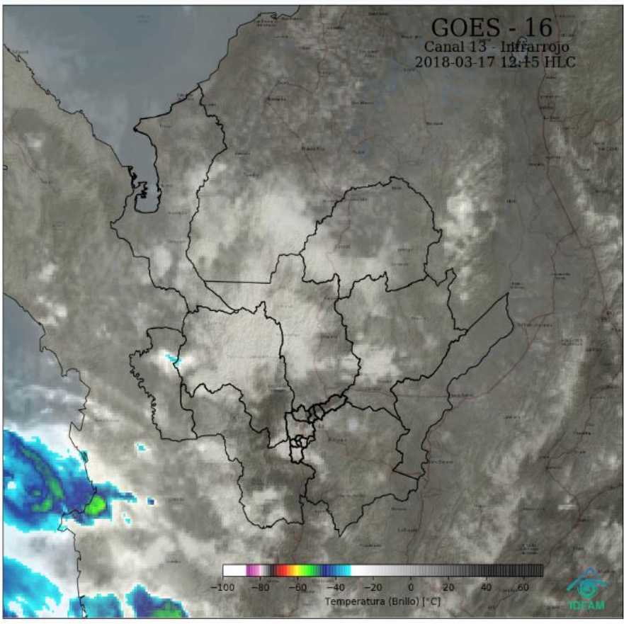
Nubosidad representada en la imagen satelital. Canal Infrarrojo – GOES 16 - IDEAM Marzo 17 de 2018 – Hora 12:15 p.m.
