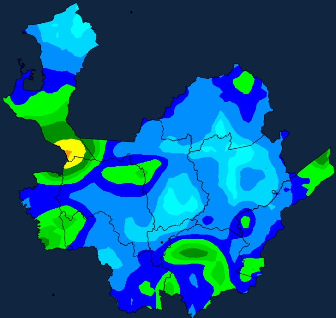
Pronóstico de precipitación acumulada en 06 horas, a partir de: 2020-10-22 18:00 HLC.
