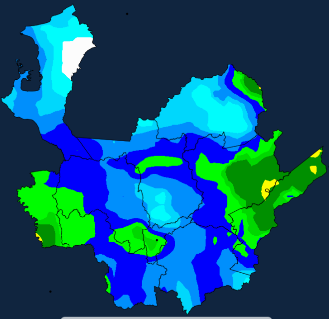
Pronóstico de precipitación acumulada en 06 horas, a partir de: 2020-10-23 00:00 HLC.
