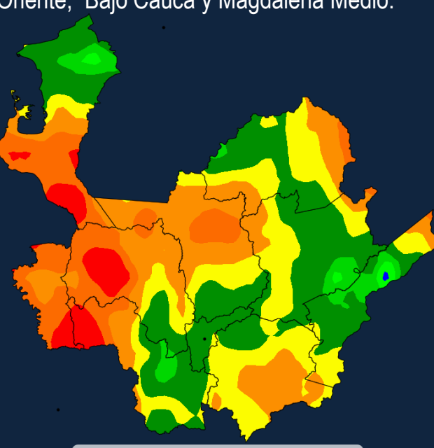
Pronóstico de precipitación acumulada 24 en horas, a partir de: 2020-10-23 06:00 HLC.
